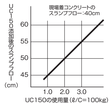
UC150の使用量とスランプフローの関係
