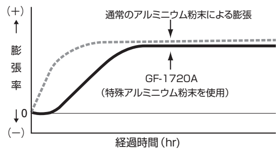
GF-1720Aの膨張概念図
