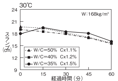
スランプの経時変化室内試験結果例
