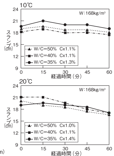
スランプの経時変化室内試験結果例
