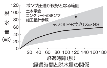
ポンプ圧送性 (加圧ブリーディング試験による評価)
